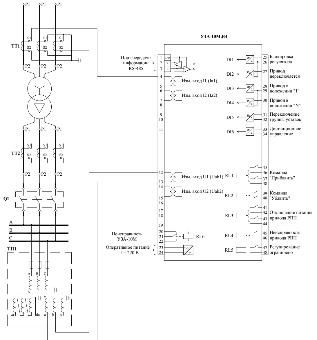
Рисунок 1. Схема подключения УЗА-10М.В4
