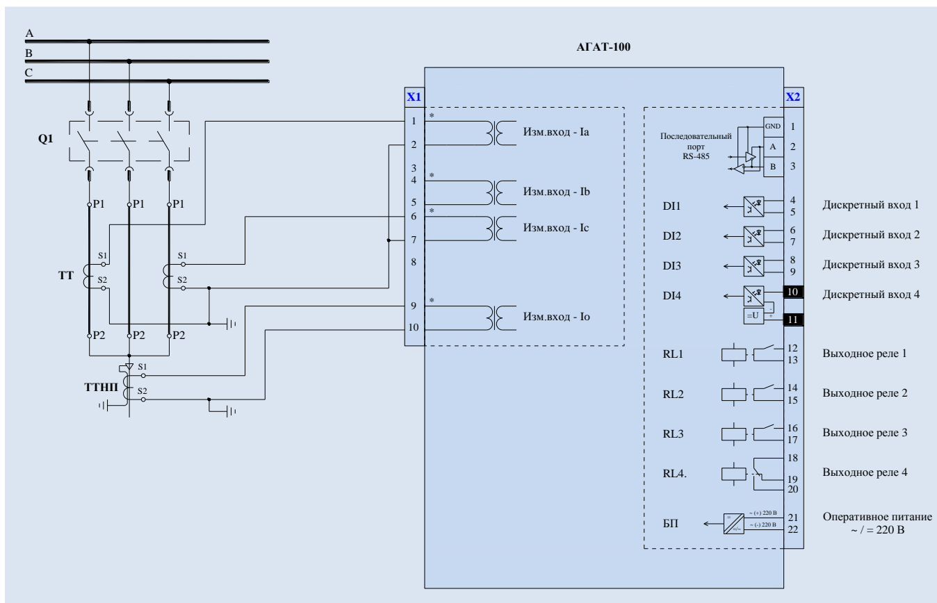
Рисунок 3. Схема подключения АГАТ-100 при использовании двух измерительных трансформаторов тока.
