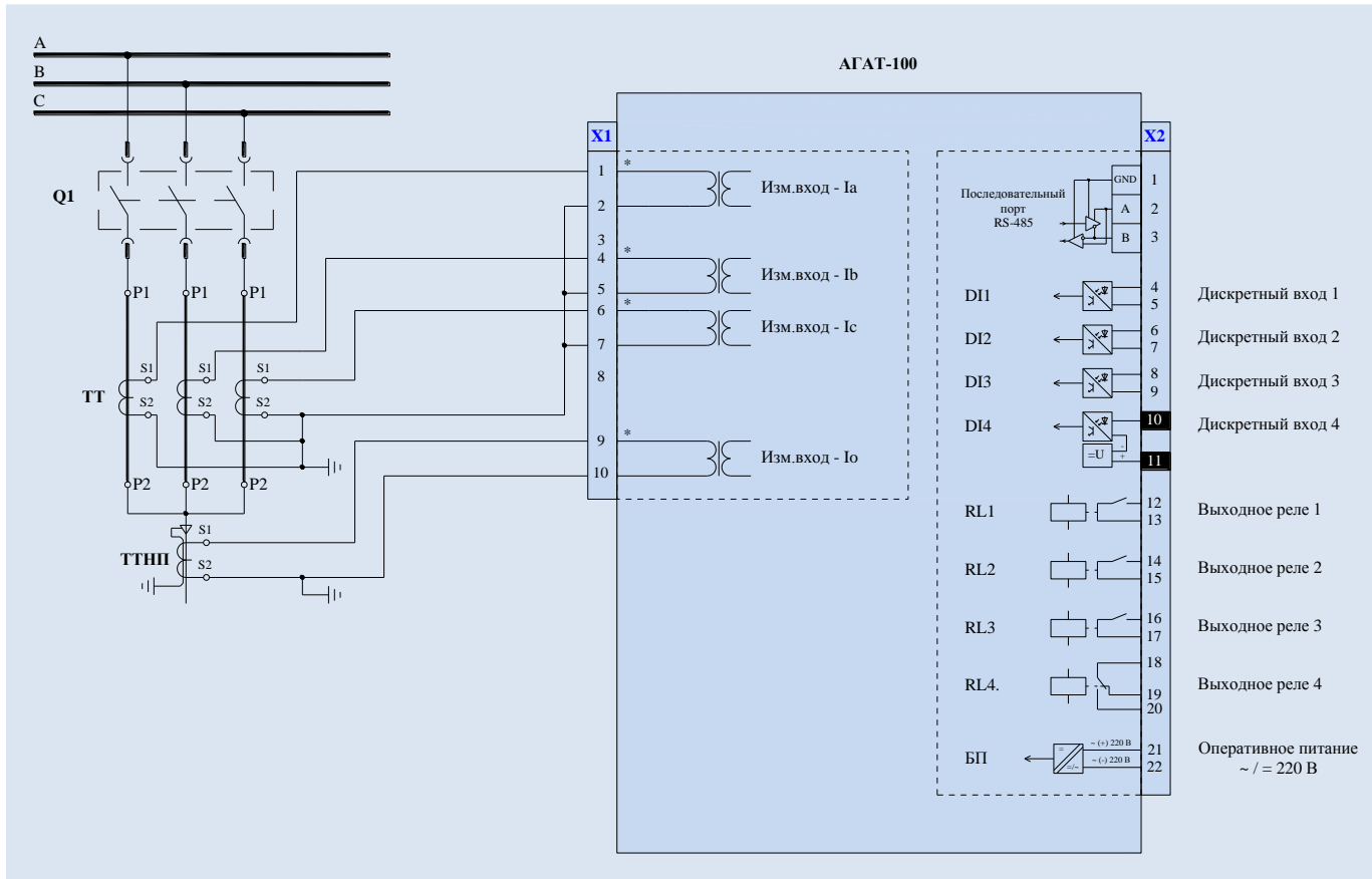
Рисунок 1. Схема подключения АГАТ-100 без выхода дещунтирования электромагнитов отключения выключателя.
