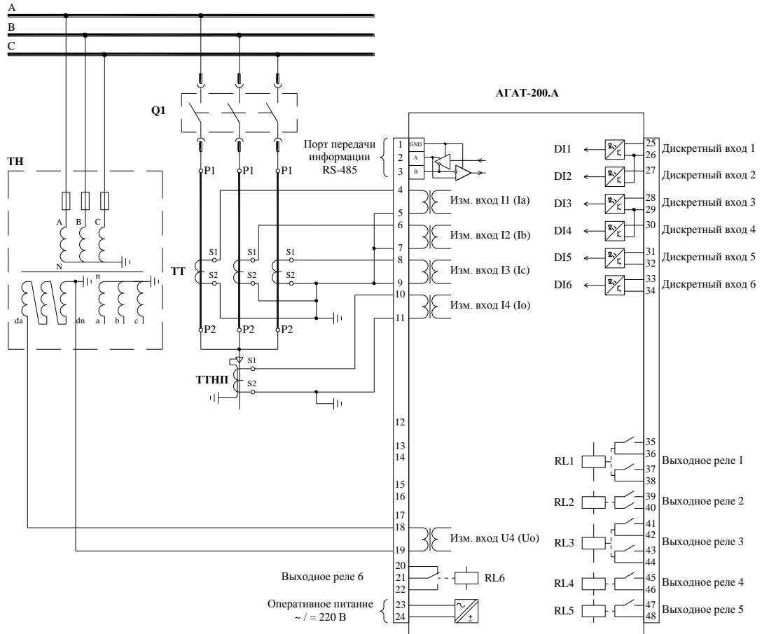
Рисунок 1. Схема подключения АГАТ-200.А с модулем входов/выходов - 6DI-6RL.
